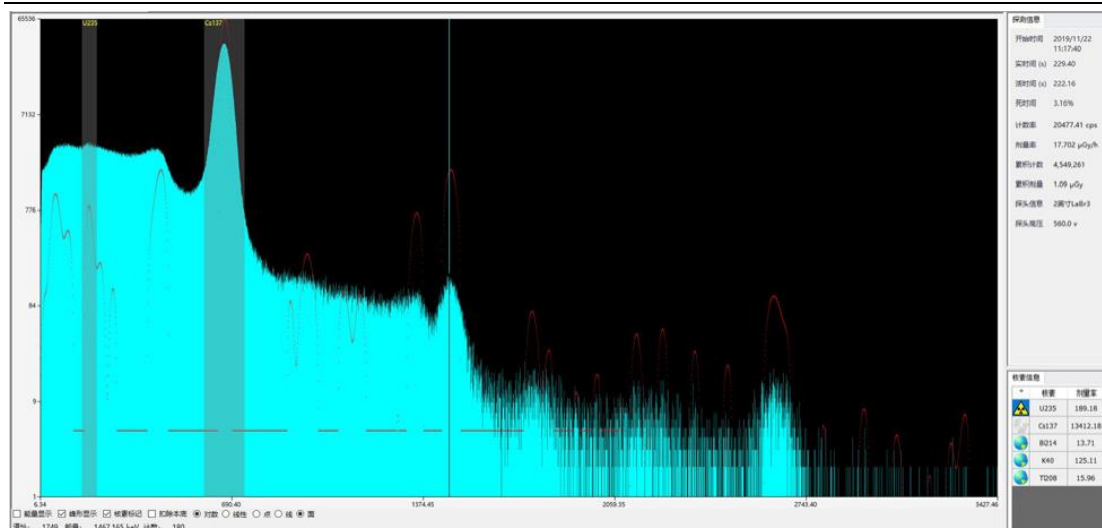
图 2 GammaArray-64 测量生成的放射性活度分布
